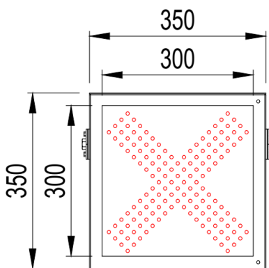
TRẠNG THÁI 1 (LÀN ĐANG ĐÓNG)
